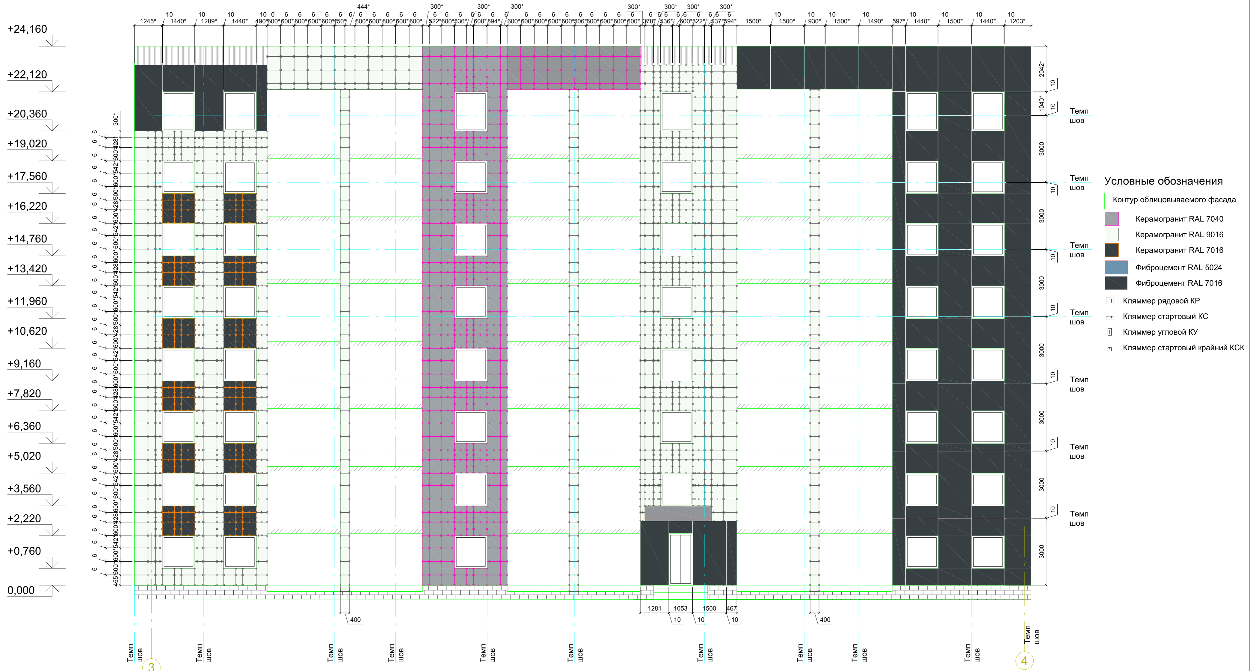
Компоновочная схема
