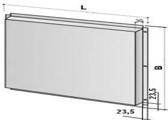
Кассета открытого крепления К-1
